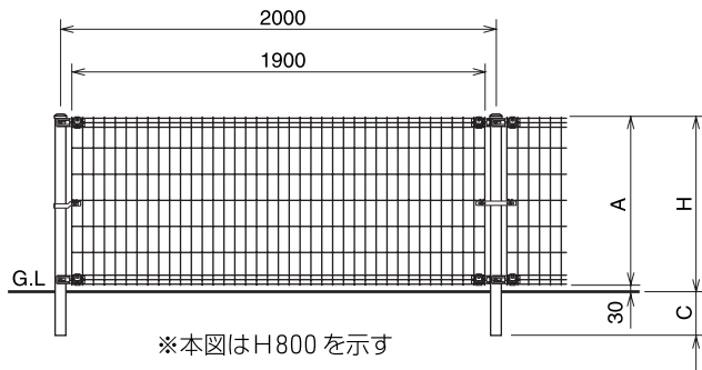
胴縁取付
